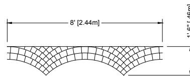
16-1-158 Top Edger
