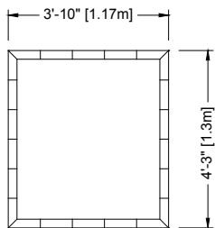
17-1-185 Signage Border
